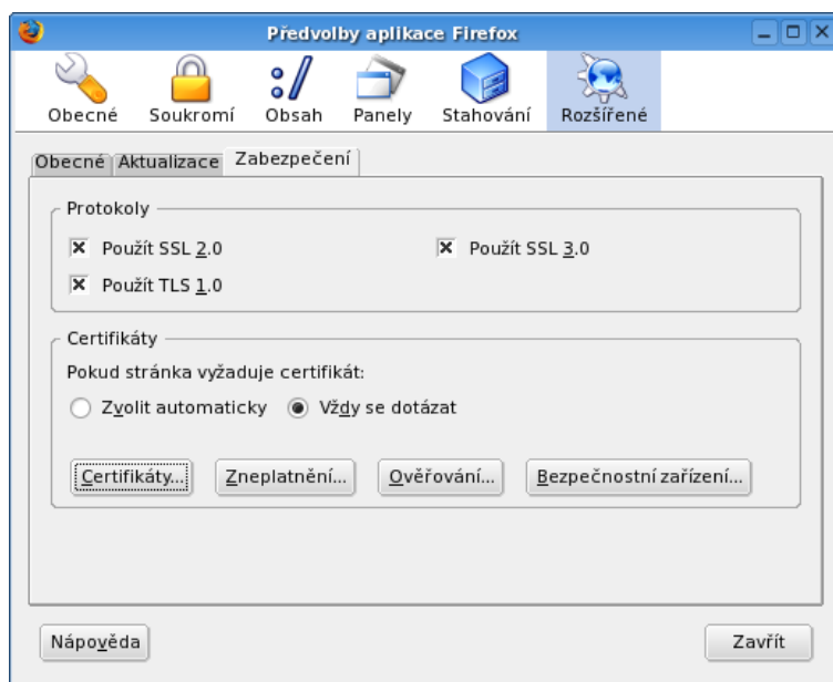
Obrázek 86: Správa certifikátů v prohlížeči Firefox (verze 1.5.0.7)
